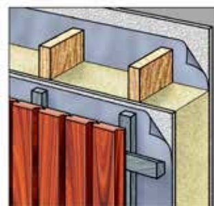
Tekening 7. Een voorbeeld van een dubbel regelwerk.
