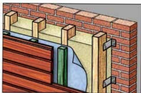
Tekening 6. Opbouw gevelbekledingsconstructie bij een steenachtig binnenspouwblad, regelwerk verduurzaamd.
